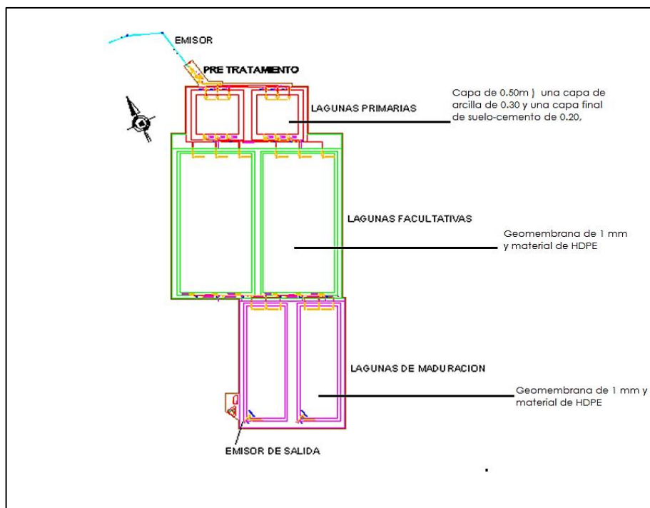
Figura 42. Distribución de las lagunas facultativas de la PTAR OMO. (Vista superior) Expediente técnico del GRM
