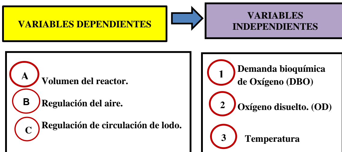
Figura 34. Relación entre las variables del controlador Elaboración propia.
