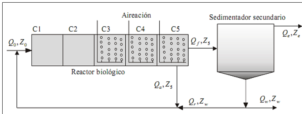
Figura 26. Esquema más detallado del proceso de flujo de lodo activado
