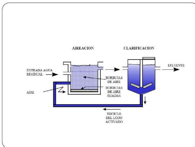
Figura 25. Esquema del proceso real, aunque sencillo, de flujo de lodo activado Recuperado de https://es.slideshare.net/ilserocio/lodos-activados?next_slideshow=1
