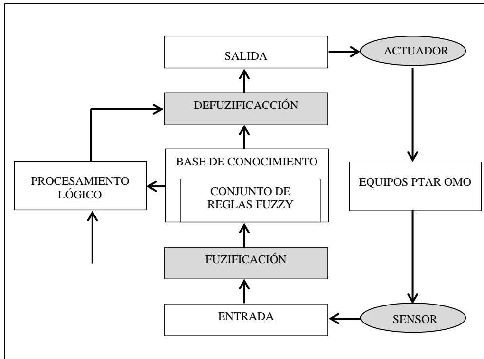
Figura 33. Figura básica de un sistema de controlador Fuzzy
