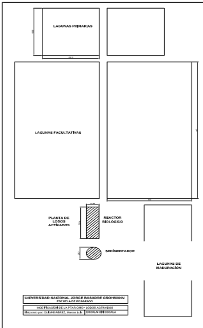
Figura 45. Propuesta de modificación de la PTAR OMO Elaboración propia
